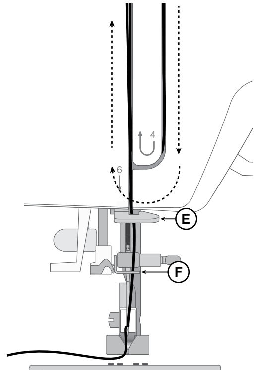
Maschine von vorne
