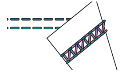
3-Faden Coverstich schmal (CC-RC)
