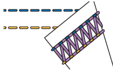
3-Faden Coverstich breit (LC-RC)
